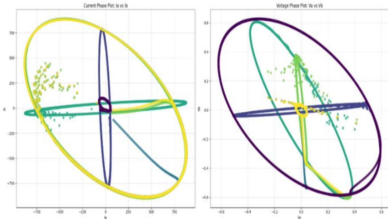
Figure 6 : Scatter plot des phases de courant et de tension ( I_a vs I_b , V_a vs V_b )
