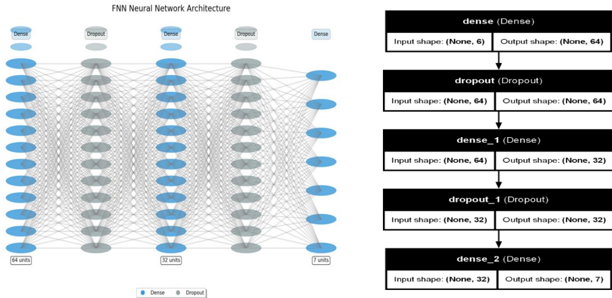
Figure 54 : Architecture et hyperparamètres – FNN
