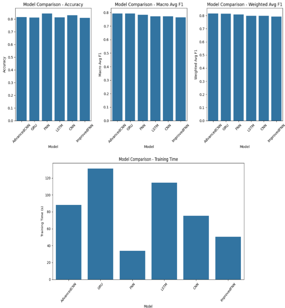
Figure 70 : comparaison détaillée des performances modèles de Deep Learning
