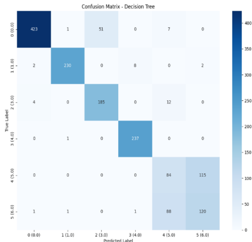
Figure 29 : Matrice de confusion
