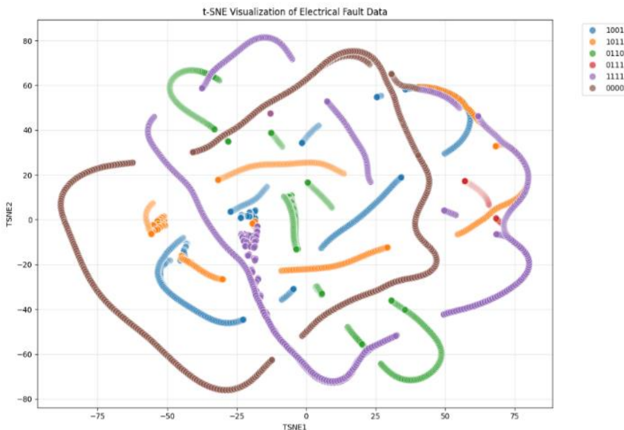
Figure 5 : Visualisation des données avec t-SNE
