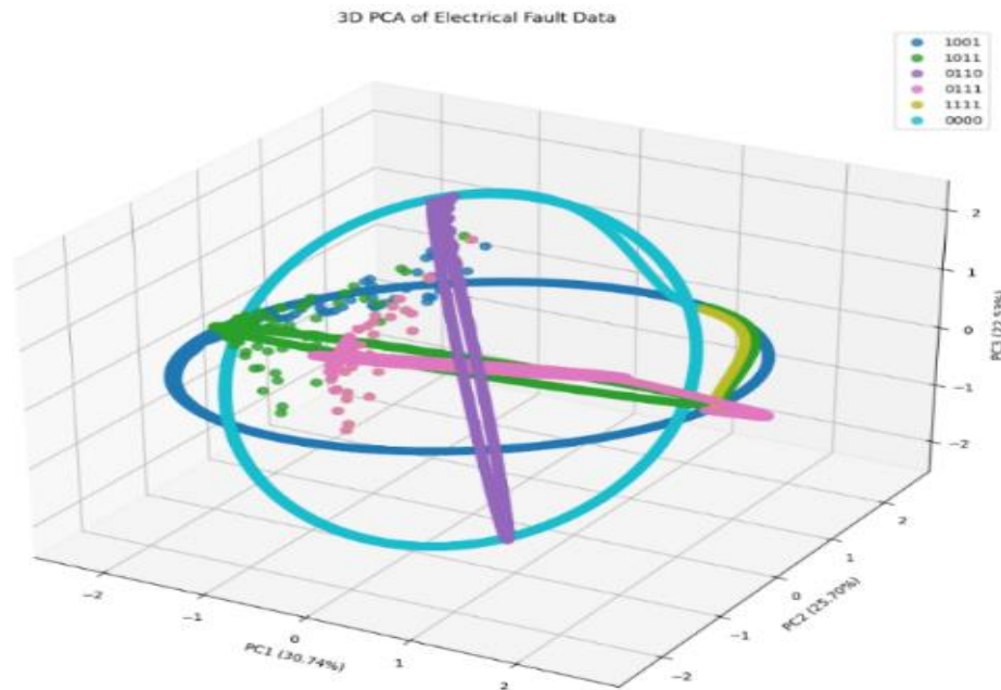
Figure 9 : Visualisation PCA en 3D des défauts électriques
