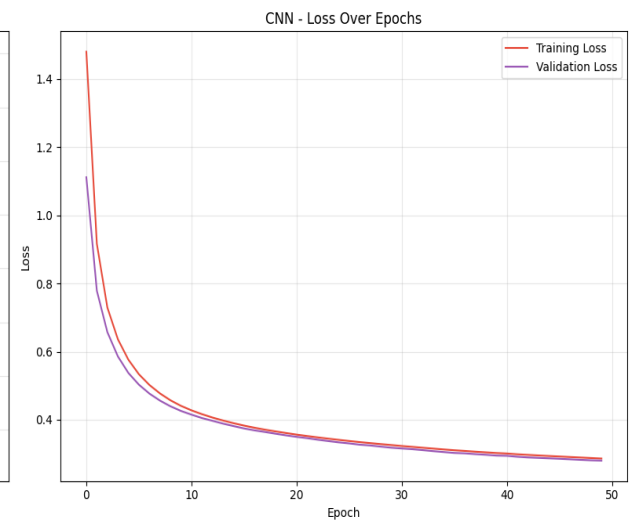
Figure 44 : Courbe d'apprentissage CNN
