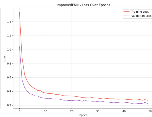
Figure 63 : Courbe d'apprentissage Improved FNN de loss over epochs
