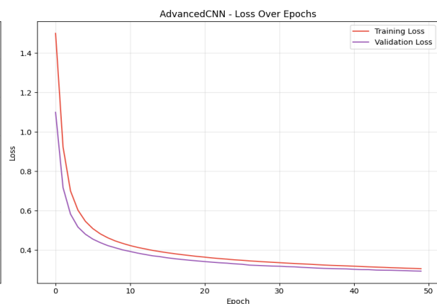
Figure 48 : Courbe d'apprentissage AdvancedCNN
