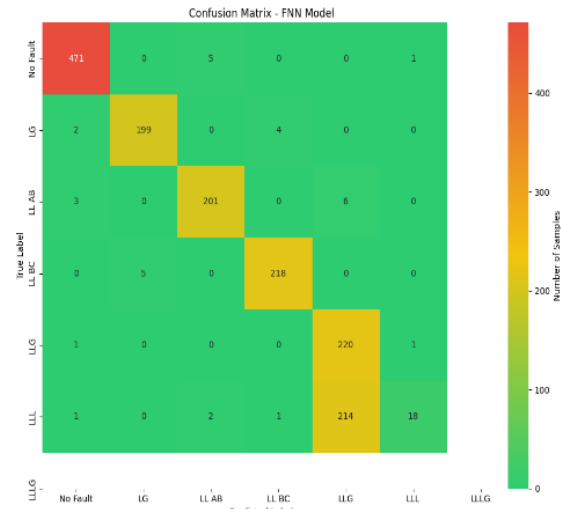
Figure 51 : Matrice de confusion de FNN evaluation
