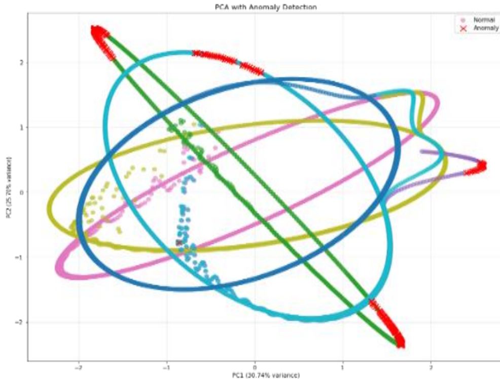
Figure 17 : Détection d'anomalies avec Isolation Forest
