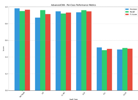
Figure 46 : F1-score par classe AdvancedCNN
