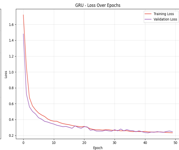
Figure 58 : Courbe d'apprentissage GRU
