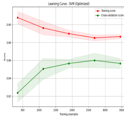
Figure 25 : Courbe d'apprentissage SVM Optimized
