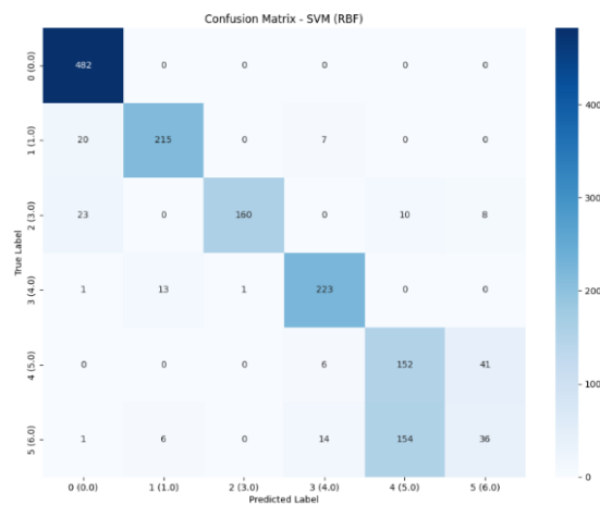
Figure 22 : Confusion de matrice SVM RBF
