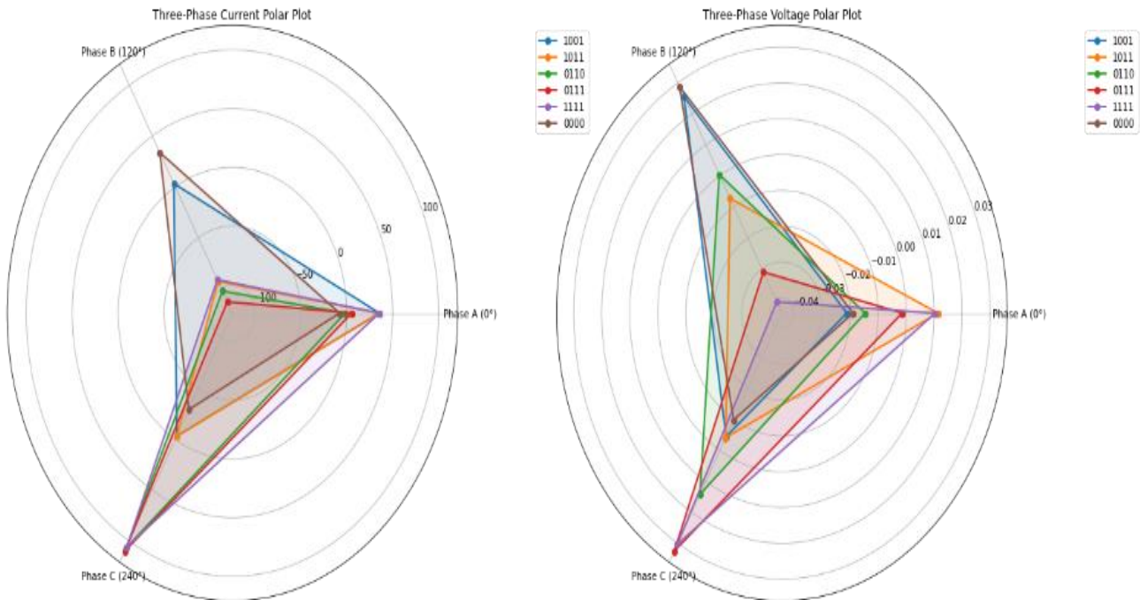
Figure 10 : Polaire des tensions et courants triphasés
