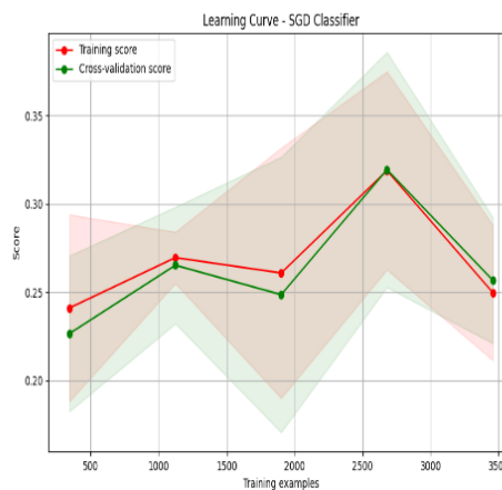
Figure 36 : Courbe d'apprentissage SGD
