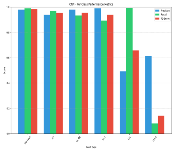
Figure 42 Déclaration de CNN Evaluation
