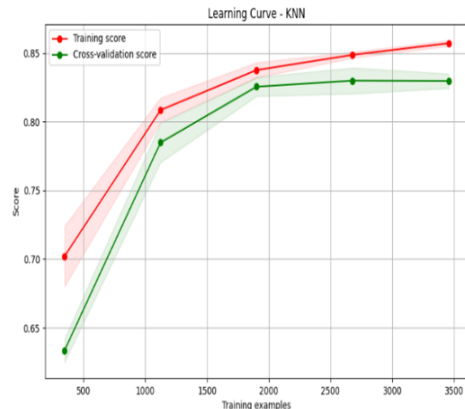
Figure 19 : Courbe d'apprentissage KNN
