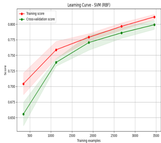
Figure 23 : Courbe d'apprentissage SVM RBF
