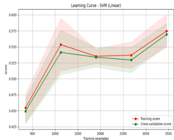
Figure 21 : Courbe d'apprentissage linear
