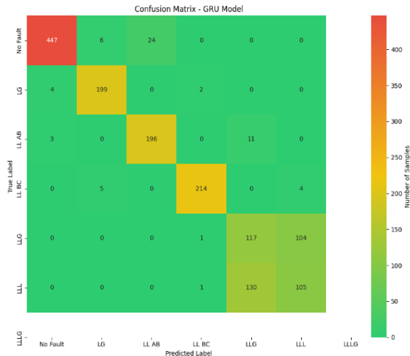
Figure 55 : Matrice de confusion de GRU
