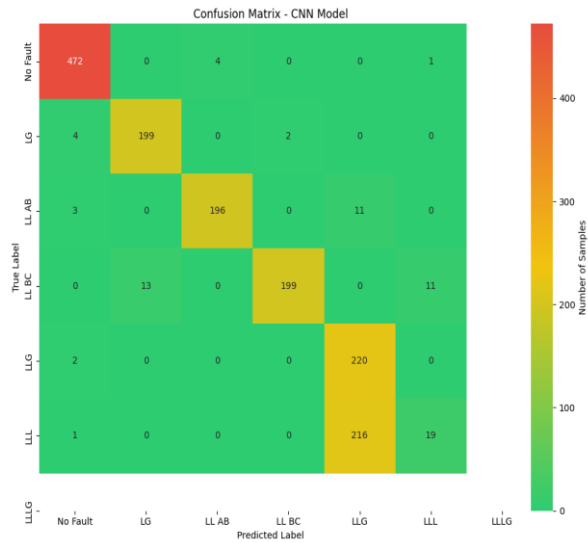
Figure 41 : Matrice de confusion
