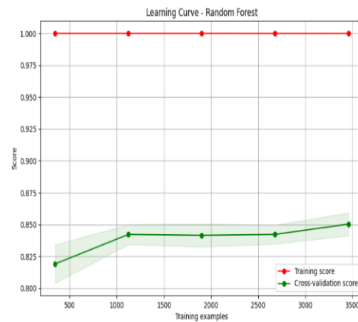
Figure 28 : Courbe d'apprentissage Forest
