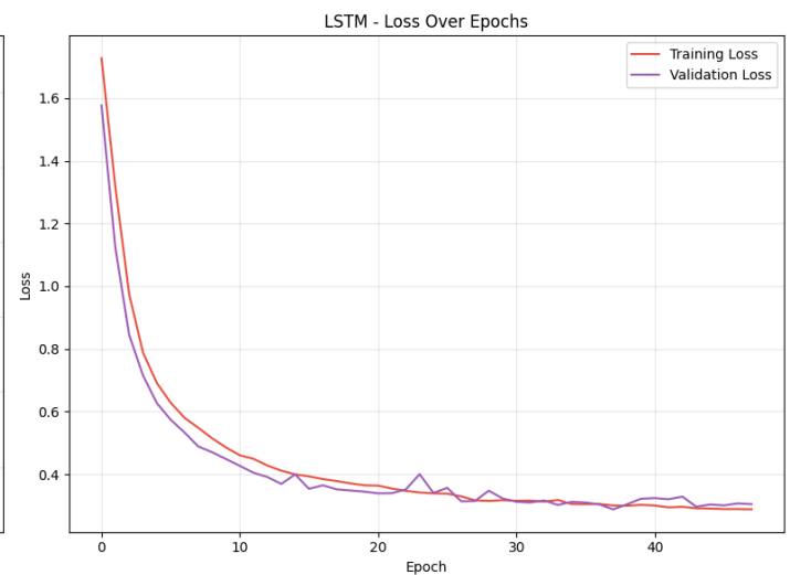
Figure 68 : Courbe d'apprentissage-LSTM Over epochs
