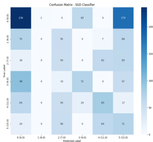
Figure 35 : Confusion de matrice SGD
