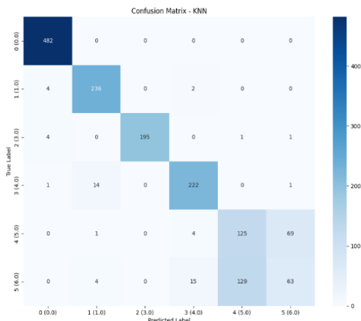
Figure 18 : Confusion de matrice KNN
