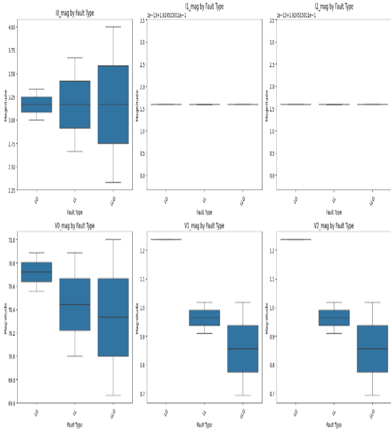
Figure 11 : Visualiser la variation de chaque composante en fonction du type de défaut
