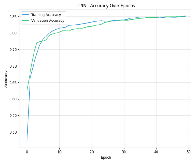
Figure 43 : Courbe d'apprentissage CNN
