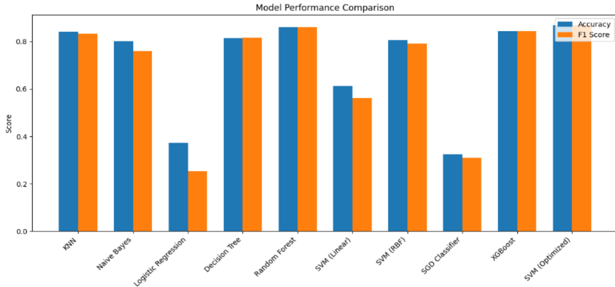
Figure 39 : Diagramme comparatif des modèles ML
