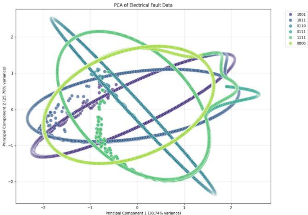
Figure 4 : Projection PCA des types de défauts
