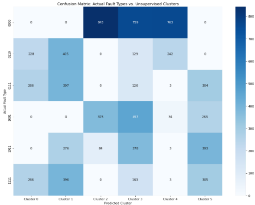
Figure 15 : Matrice de confusion pour le clustering non supervisé
